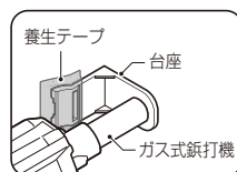
①ガス式鉸打機で台座を固定します。
