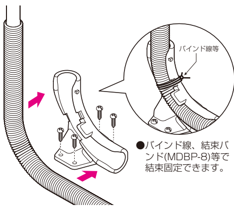
スリーブ 材質：PP
