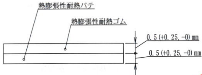
耐火シート (樹脂メッシュ無) の断面図
