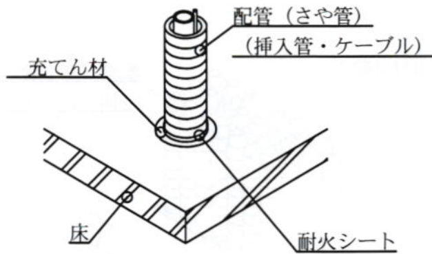
円形開口の場合 (単配管)
