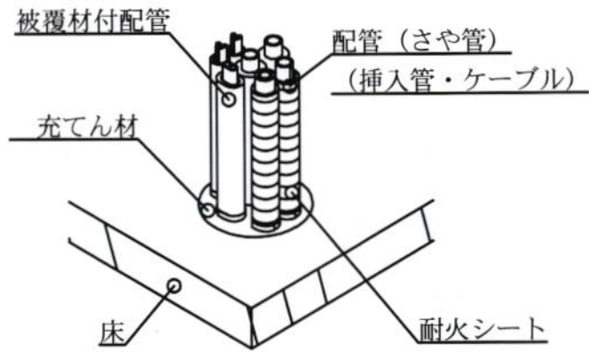
円形開口の場合
