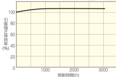
■ 使用材料のサンシャインウエザオメーターテストによる引張強さ変化 (ブラックパネル温度83°C、雨なし)
