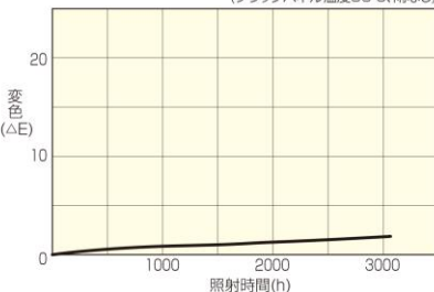
■ 使用材料のサンシャインウエザオメーターテストによる色変化 (ブラックパネル温度83°C、雨なし)
