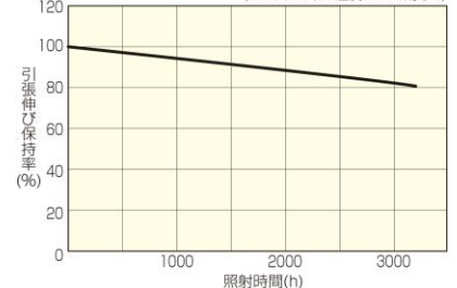
■ 使用材料のサンシャインウエザオメーターテストによる引張伸び変化 (ブラックパネル温度83°C、雨なし)
