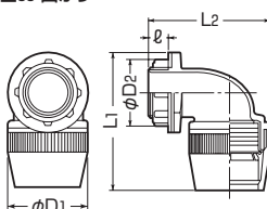
■90°曲がり
