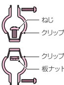
取付方法
