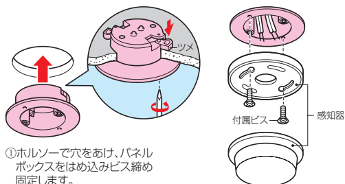
(弱電用) SBP-K 取付ボード厚 (3~18mm迄)
