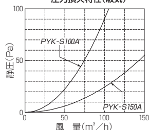
圧力損失特性(吸気)
