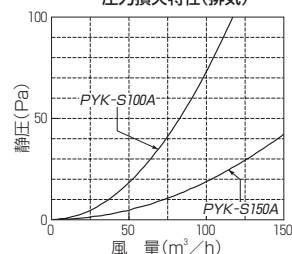
圧力損失特性(排気)
