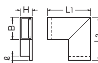
■1010・715・1020・1025・1030型
