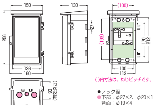
■WB-3A□ ●木板ベース付●バンド通し穴：側面
