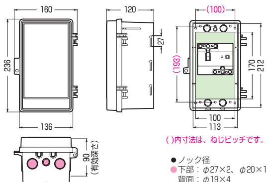
■WB-3AO□ ●木板ベース付●バンド通し穴：側面
