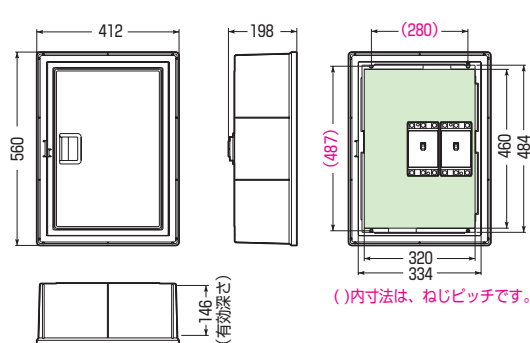
■WB-5AO□ ●木板ベース付
