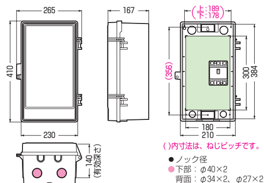
■WB-5AO□ ●木板ベース付
