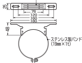
■POB-2型 器具取付溝(有効深さ20mm)
