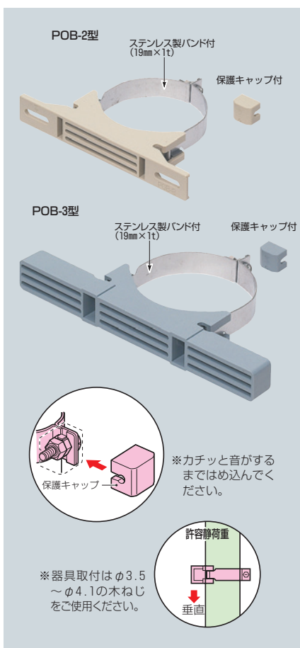
■POB-2型 器具取付溝(有効深さ20mm)
