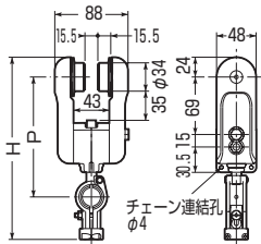
メインローラー ベアリング仕様
