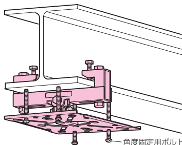
角度固定用ボルト
