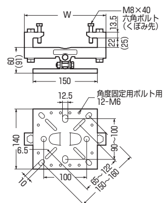
角度固定用ボルト
