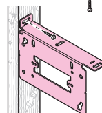
■垂直柱への取り付け
