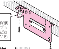
■ボックスを使用しない取り付け
