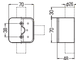
底面ノックアウト：φ22・16(19)×1
