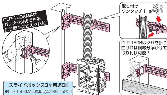
■CLP-150B
