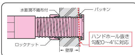
ジョイントGPアダプター付2号コネクタ
