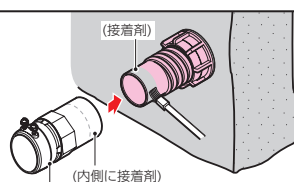
ジョイントGPアダプター付2号コネクタ
