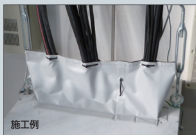
■2列間カバー
