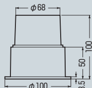
固定ブロック(ポイントタイプ) スペーサー
