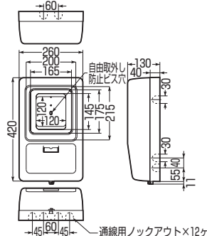
WP-2W型
