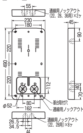
■BP-3L型
