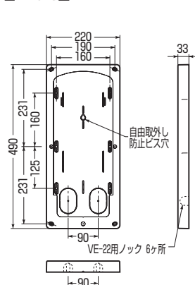
■BP-3LS型
