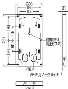
■BP-3L型
