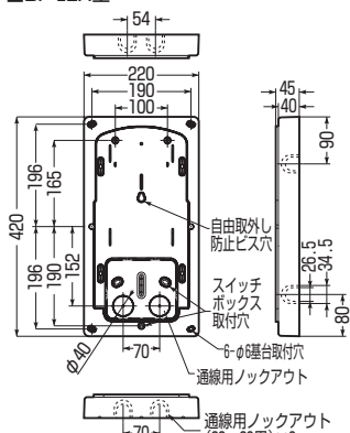
■BP-3LS型
