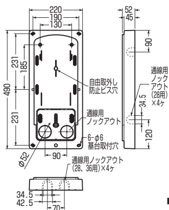
■BP-3LH型
