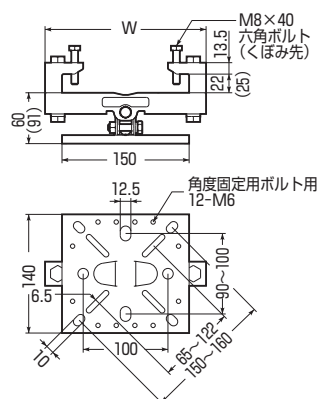
角度固定用ボルト
