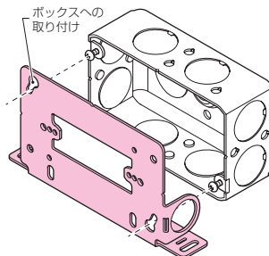
■当社スライドボックス1個用への取り付け
