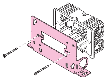
■当社スライドボックス1個用への取り付け
