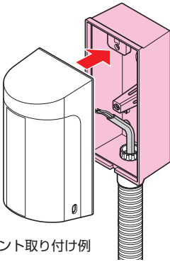
■PVR22-LBCJ
