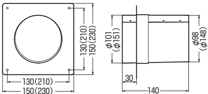
0.5mm厚 ※ ( )内寸法はPYSB-S150です。
