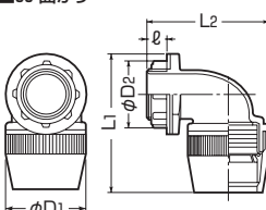
■90°曲がり
