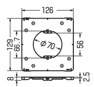
■丸型(平)
