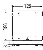
■プランク(平)
