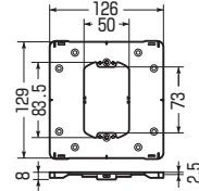
■小判型(平)
