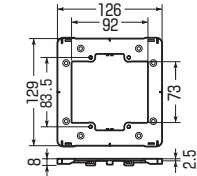
■2個用(平)
