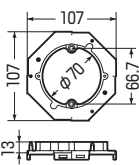
■丸型(塗代付)
