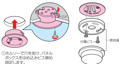
(弱電用) SBP-K 取付ボード厚 (3~18mm迄)
