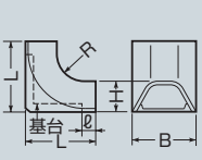
■立上げ
