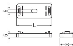
■VP台付サドル用スペーサー
