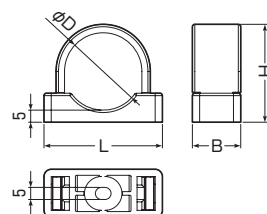
■VP台付サドル用スペーサー
