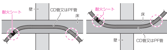
■サブウェイ工法(KK26-010号)
