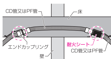
■サブウェイ工法(KK27-015号)
