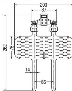
■FLB-T4570
