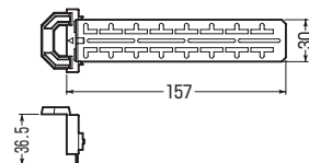
■CLP-150KMA
