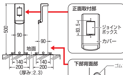
アース用 ねじ・座金付
