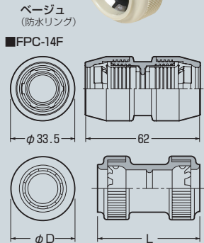
FPC-14F (内部バッキン)
