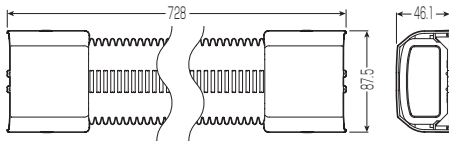
専用ソケット2ヶ付
