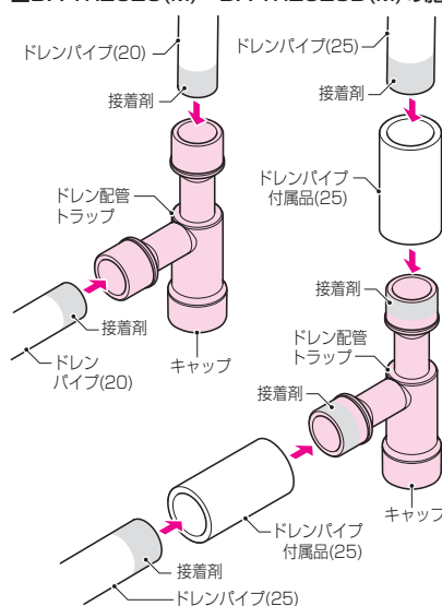
■20サイズを配管する場合
