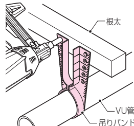
■根太に固定する場合
