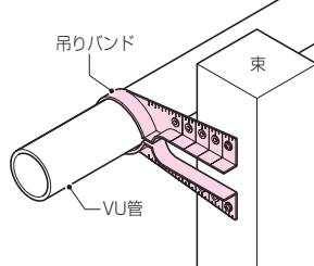
■束に固定する場合
