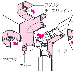
●樹脂管
