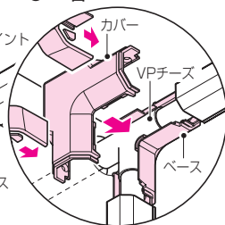
●VP管
