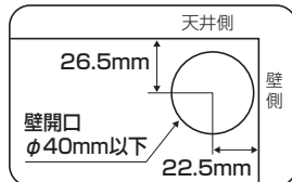
壁開口位置
