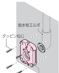
給水栓用ボックス(ベース)
