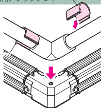
16 配管用アタッチメント
