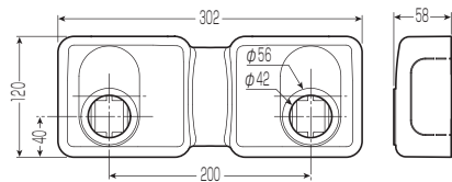
1620スペーサー
