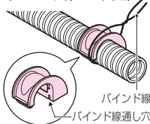
〈バインド線での固定〉
