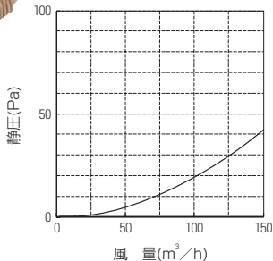
圧力損失特性
