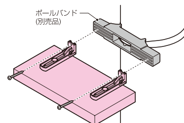
■ポールに取り付ける場合
