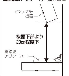
■電磁波アブソーバー取付位置
