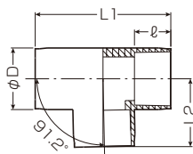
■チーズ
