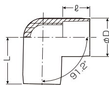
■エルボ
