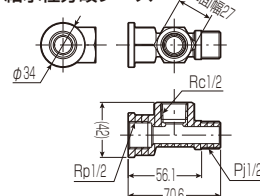
給水栓分岐チーズ
