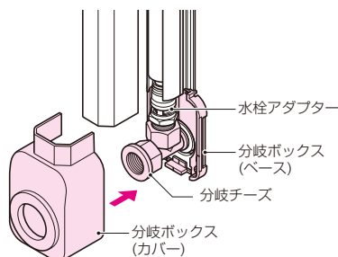
給水栓分岐チーズ
