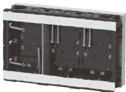
SBG-S3WO-DBF (セパレーター付)
